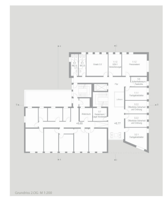
Grundriss 2.OG M 1:200
